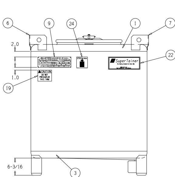
LEFT SIDE
